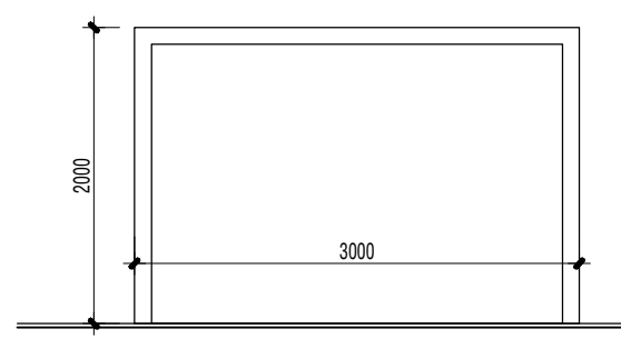
MẶT ĐỨNG KHUNG THÀNH
