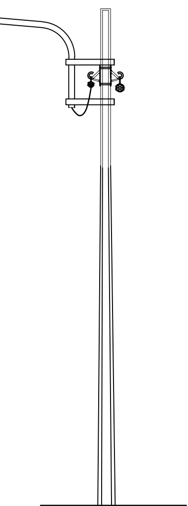
CHI TIẾT TRỤ ĐÈN
