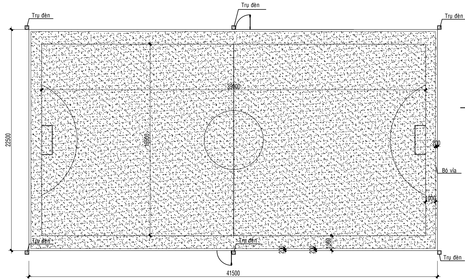
MẶT BẰNG SÂN BÓNG ĐÁ MINI (TL: 1/50)
